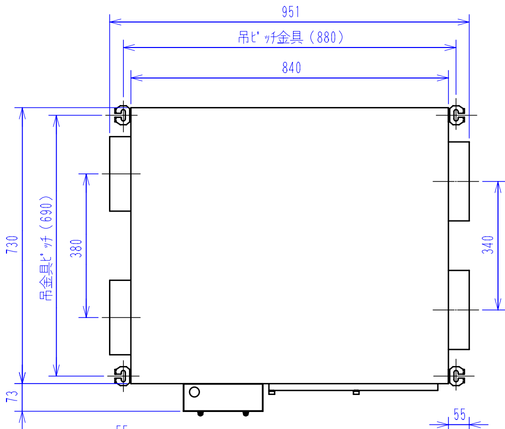
HG321D外形図
