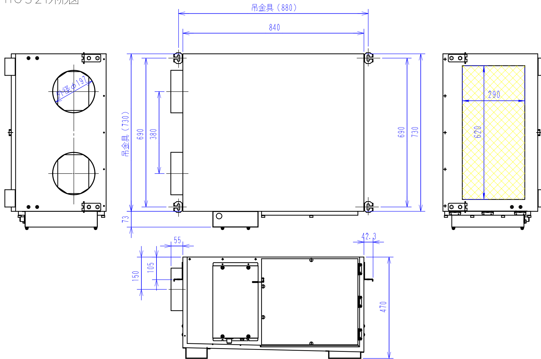
HG 321外形图
